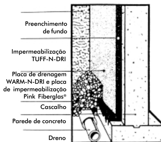
Figura 3. Exemplo de um sistema de impermeabilização para fundações.
