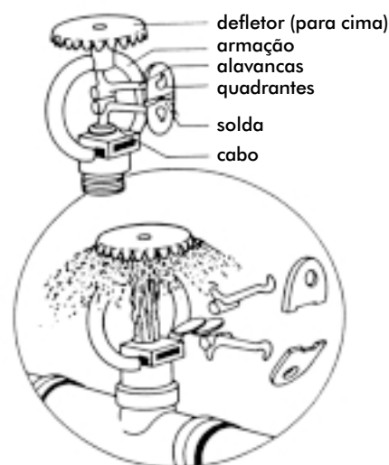
Figura 8. Cabeça aspersora típica em posições fechada e aberta (adaptado de Wayne G. Carson e Richard L. Klinger, Fire Protection Systems , 1986, National Fire Protection Assoc.)
